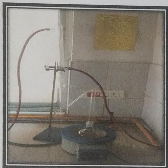
Clevenger Apparatus
