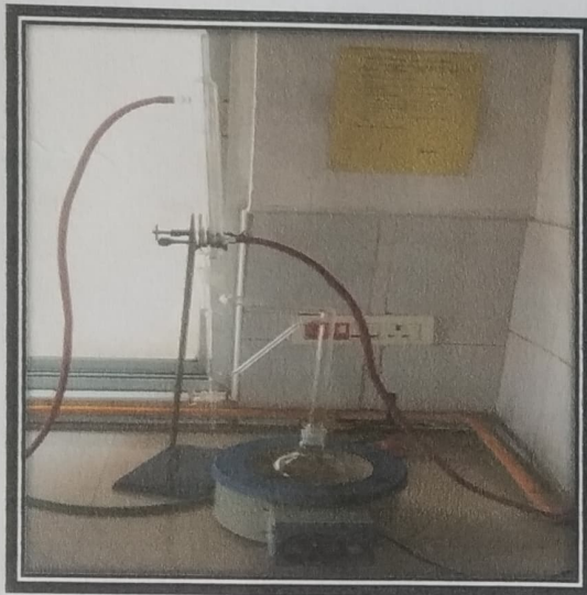
Clevenger Apparatus
